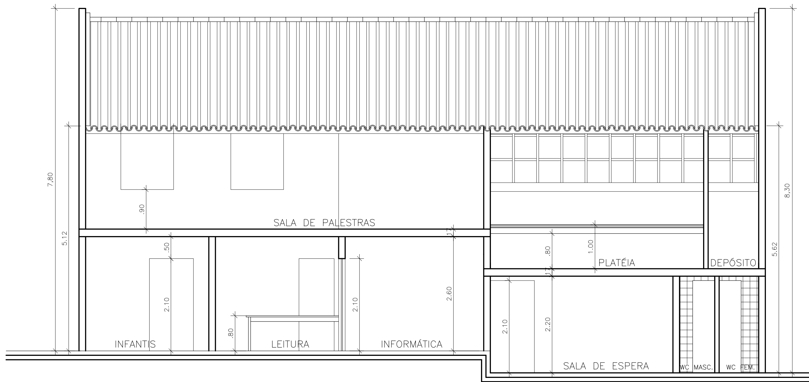
CORTE - BB
